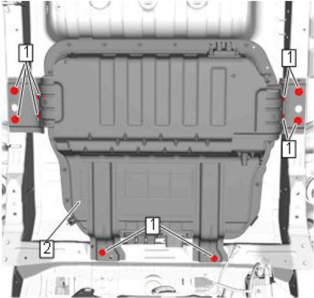
附件 1： 电池包位置示意图
